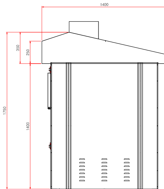
측면 VIEW
