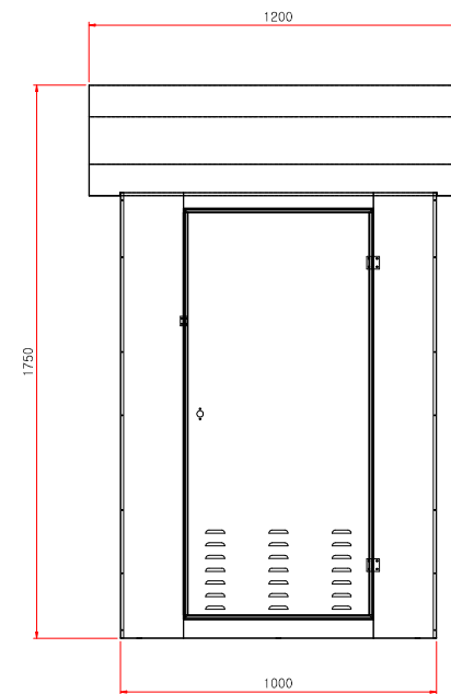
후면 VIEW
