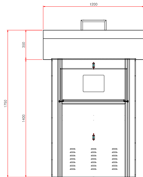
전면 VIEW
